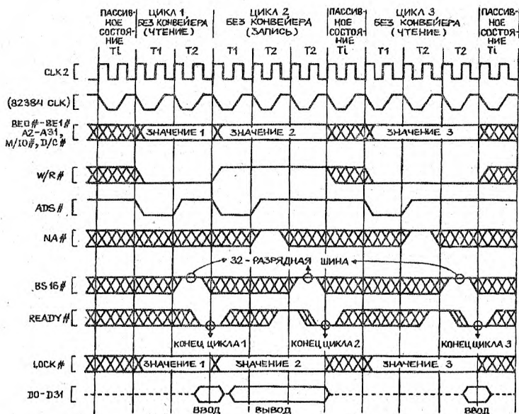
Рис.2.7. Циклы с тактами ожидания
