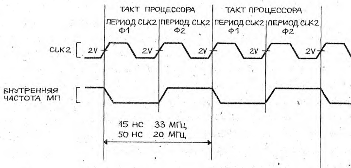
Рис.2.3. Синхросигнал CLK2
