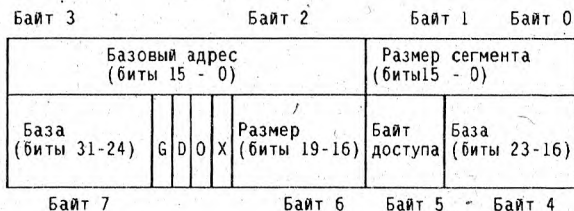
Рис. 5.3. Общий формат дескриптора
