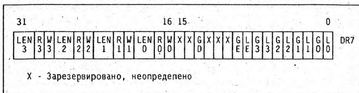
Рис. 7.2. Формат регистра DR7.
