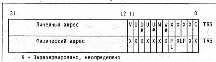
Рис. 7.1. Формат регистров TR6 и TR7
