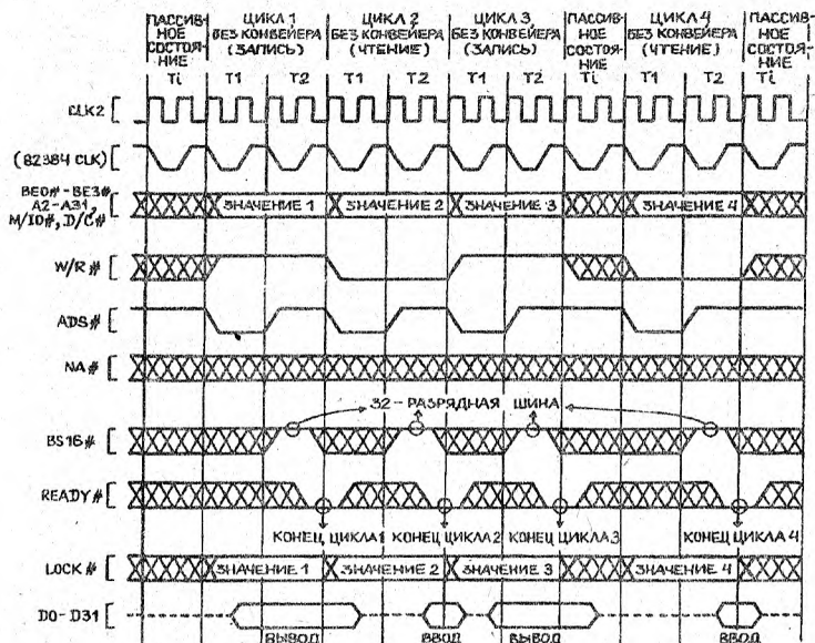
Рис.2.6. Циклы без тактов ожидания
