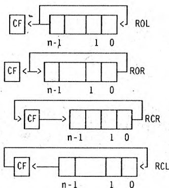
Рис.4.1. Выполнение команд циклических сдвигов
