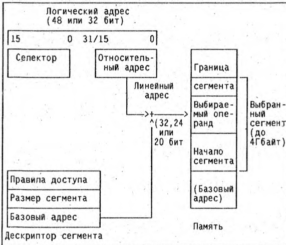
Рис. 5.2. Формирование линейного адреса
