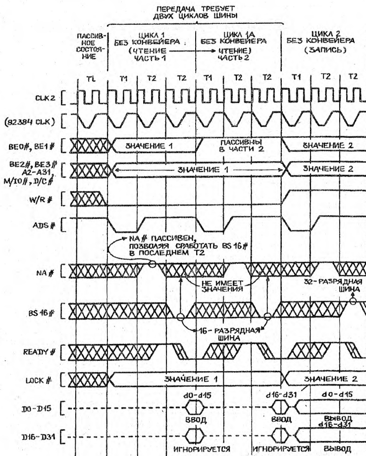
Рис.2.10. Обмен по 16-разрядной шине (с тактами ожидания)
