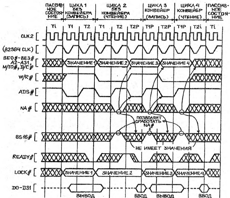
Рис.2.11. Переход к конвейеру адресов
