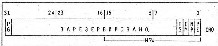
Рис.1.5. Регистр управления CR0
