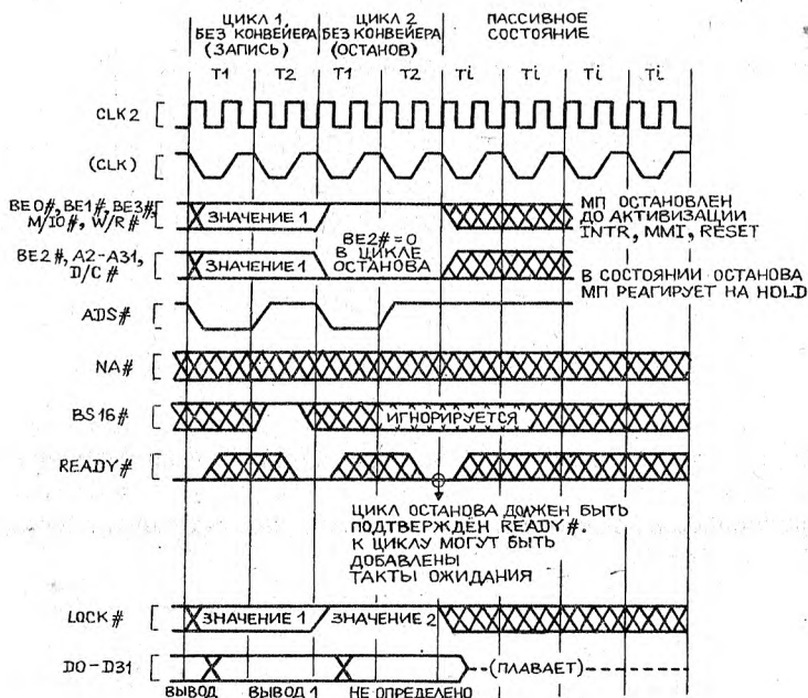
Рис. 2.16. Цикл индикации останова
