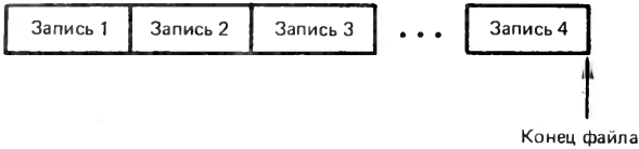
Рис. 2. Структура файла с последовательной организацией
