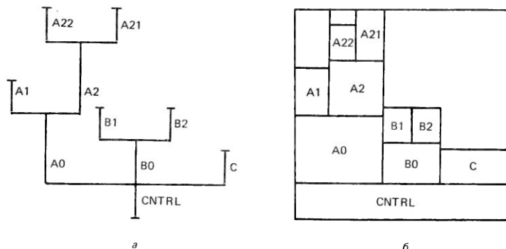
Рис. 7. Структура задачи с перекрытиями: а — дерево перекрытий для задачи; б — диаграммы распределения памяти
